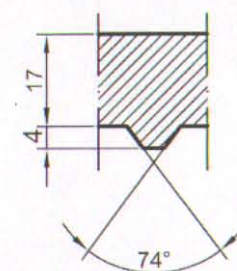
Delimičan presek B - B
