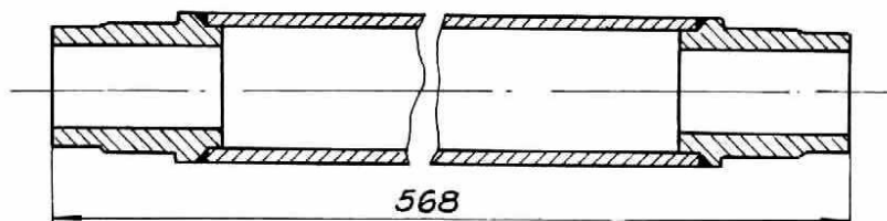
SKLOP LEŽIŠTA 2
