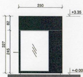
леви бочни изглед
