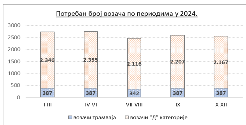
Слика 3.3.2. Потребан број возача по периодима у 2024.
